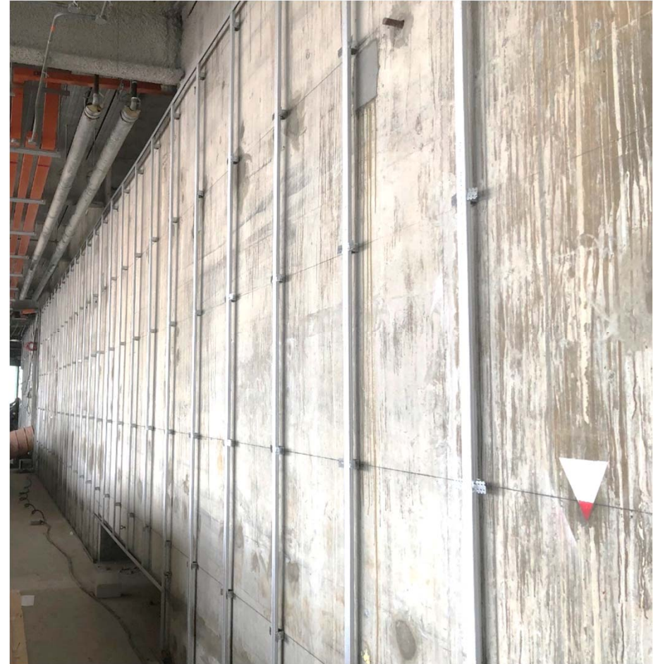
Drywall cladding
